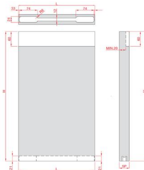
Medidas puerta de madera
