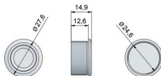
Fingerprint module / Fingerpint Modul
